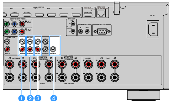
本机（后部）
